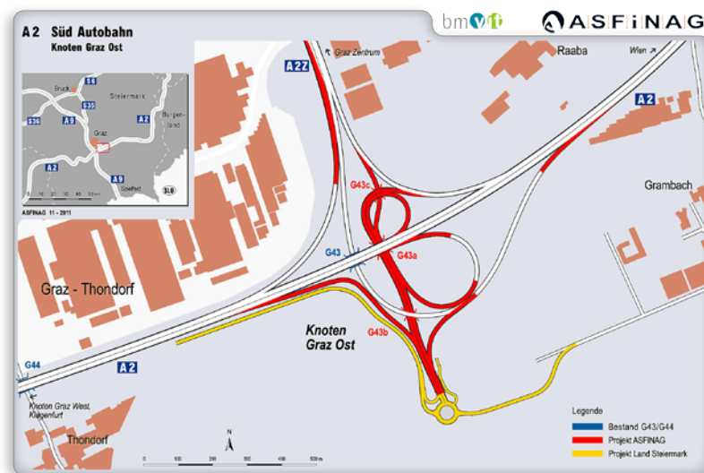
So wird der fertige Knoten Graz-Ost aussehen.
